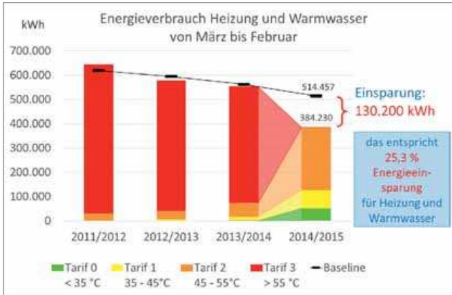
Optimierung der Rücklauftemperatur führt zu günstigeren Fernwärmertarifen, geringeren Anschlusswerten & höherem Wirkungsgrad.
